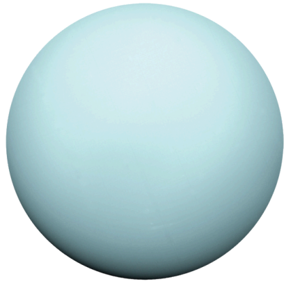
Uranus
